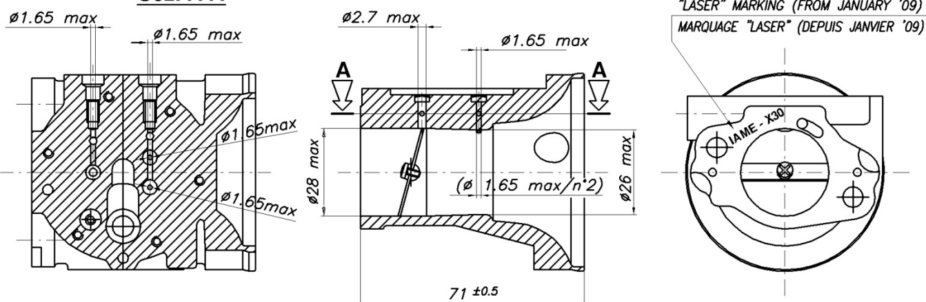
Sez. A-A
